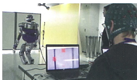
脳波によるヒューマノイドコントロール
